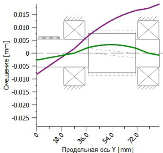
Рис. 3. Деформация вала
