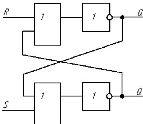
Рис. 5. Схема асинхронного RS-триггера на элементах «2 ИЛИ-НЕ»
