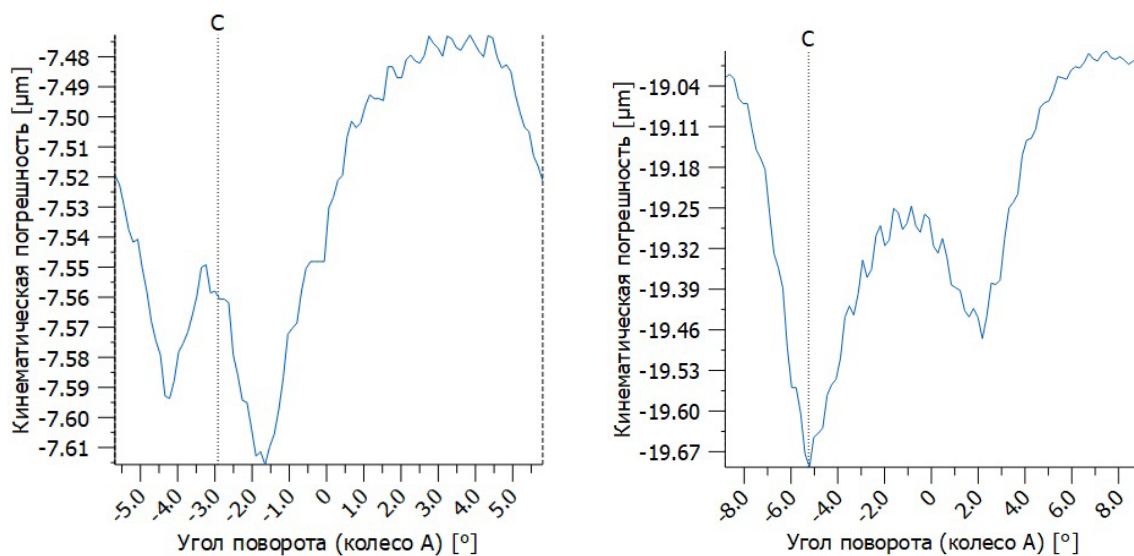
Рис. 12. Ошибки передачи на шестернях быстроходной и тихоходной ступеней
