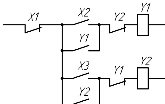
Рис. 2. Управляющая цепь
