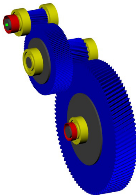
3D-модель редуктора.
